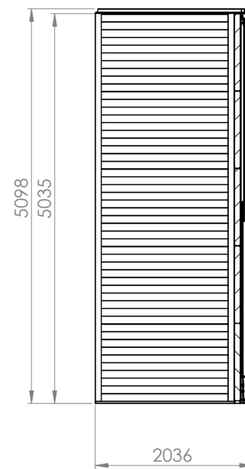
SECTION A-A
